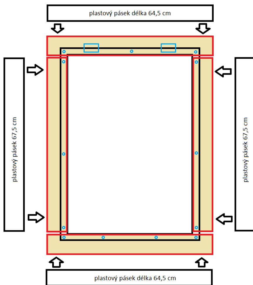
Obrázek 3 – umístění šroubů
